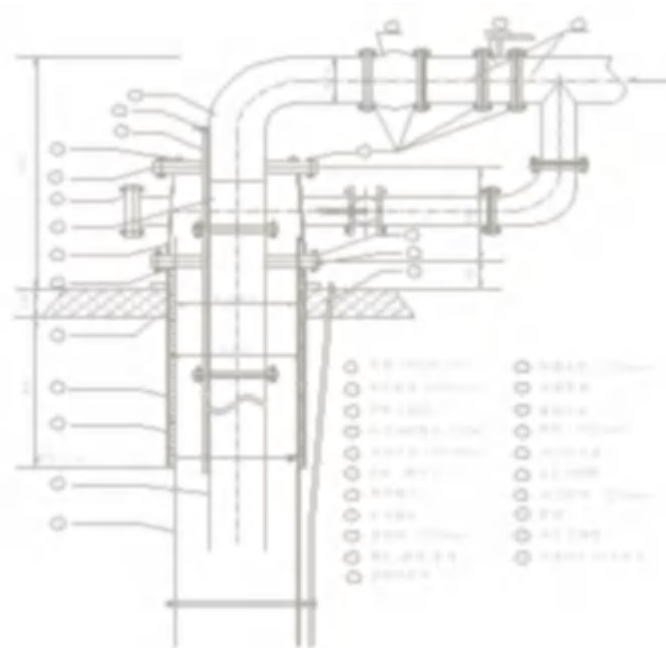
图 1-9 地热井标准井口装置基础设施图
